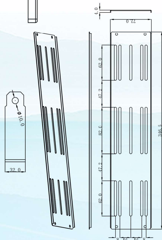
电源板孔位
